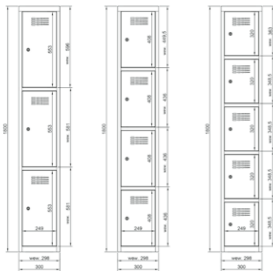
Schließfachbreite 30 cm
